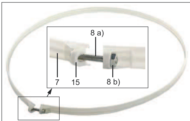
Fig.40: Montaggio nastro di fissaggio
