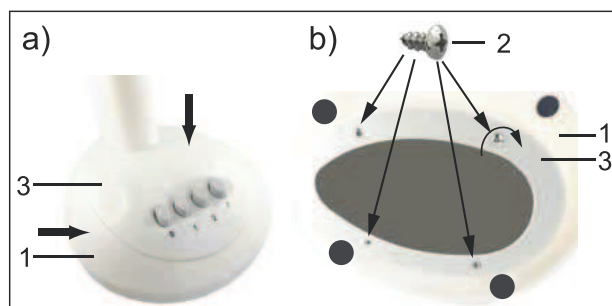
Fig.25: Montage de la base
