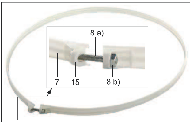
Fig.52: Montaje de la cinta de fijación
