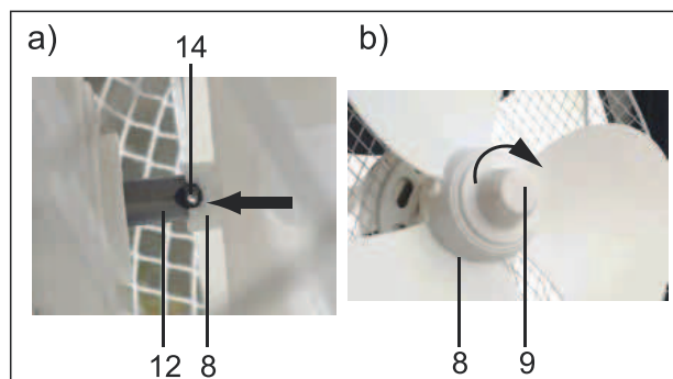
Fig.27: Montage du rotor
