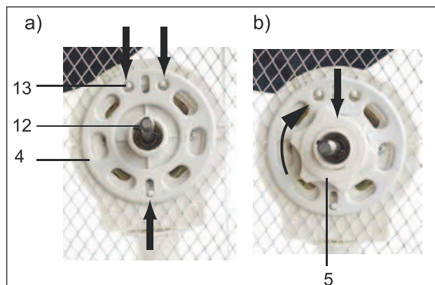
Fig.26: Montage de la grille protectrice arrière
