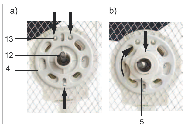
Fig.50: Montaje de la rejilla de protección trasera
