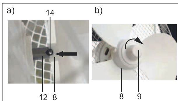
Fig.51: Montaje del rotor
